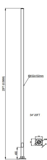
S4-20FT
