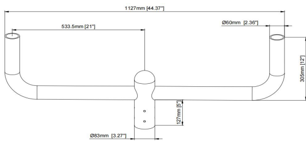
SU-SB-ACC-AL-1
