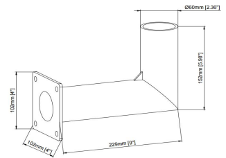
SU-SB-ACC-AL-3
