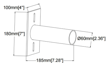
SU-SB-47R1-BR
