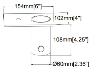
SU-SB-46R1-BR
