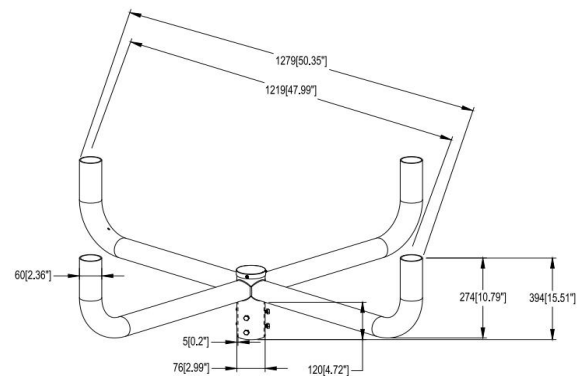
SU-SB-ACC-AL-6
