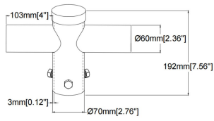
SU-SB-2.7R2-BR
