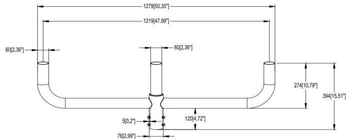
SU-SB-ACC-AL-4
