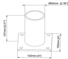
SU-SB-ACC-AL-2
