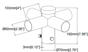
SU-SB-2.7R4-BR
