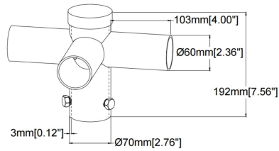
SU-SB-2.7R3-BR
